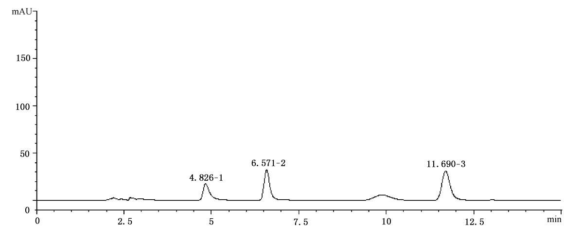
b) 加标样品液相色谱图
