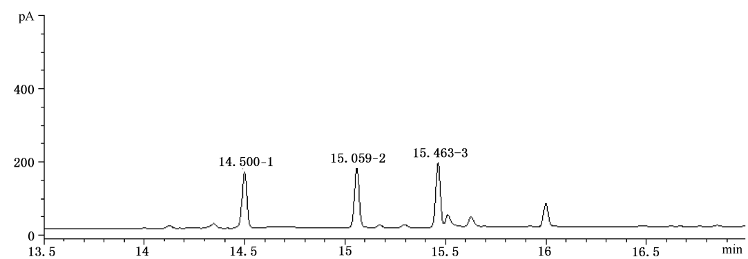
b) 加标样品气相色谱图
