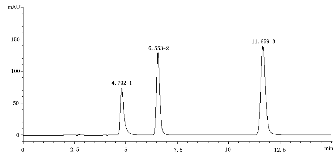
a) 标准物质液相色谱图
