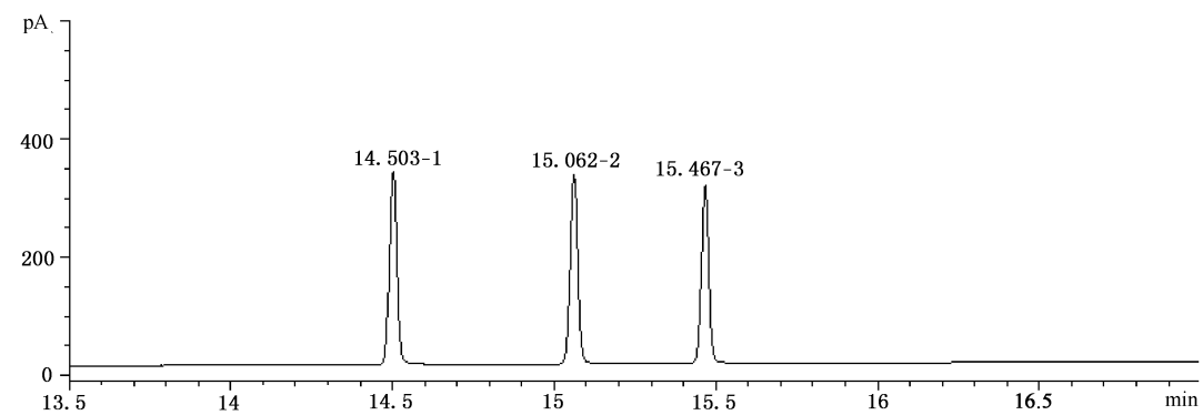
a) 标准物质气相色谱图
